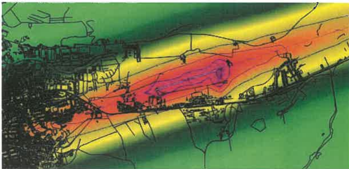
Cartare Zgomot Aeroportul Internațional Cluj– Indicator L 50 / predicție pentru anul 2017 cu distribuția reală a mișcărilor de aeronave
