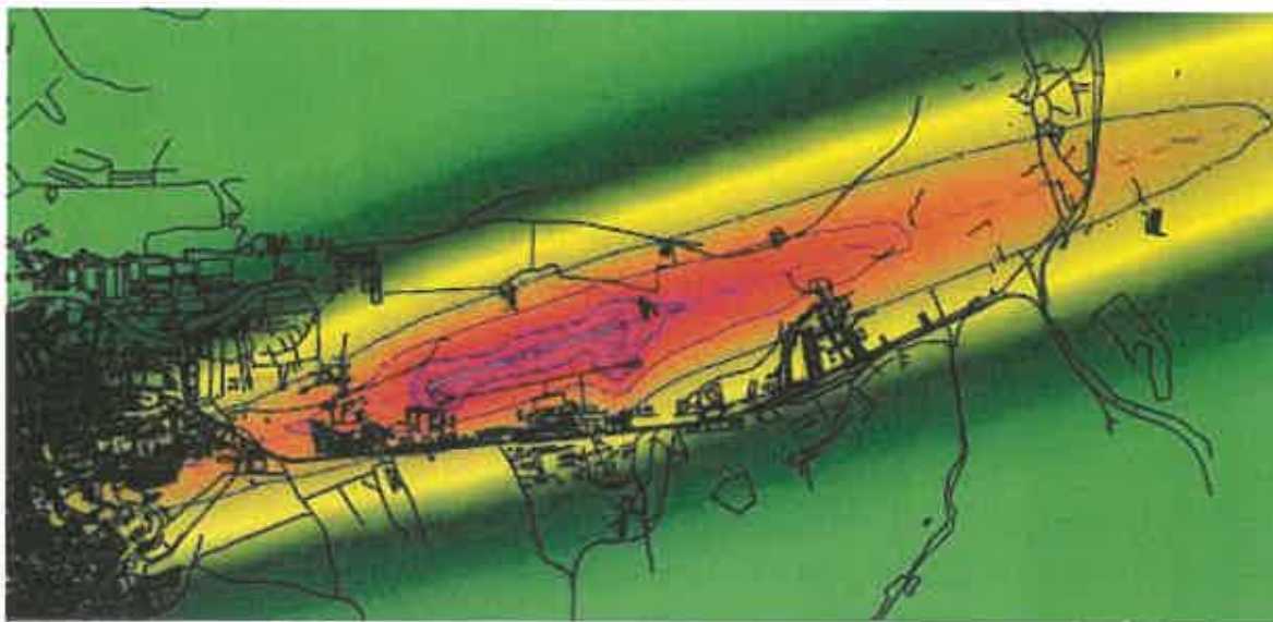
Cartare Zgomot Aeroportul Internațional Cluj – Indicator L_{ZSM} / predicție pentru anul 2017 cu distribuția mișcărilor de aeronave conform anului 2014
